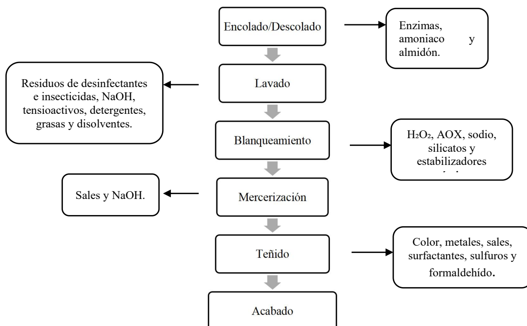
Figura 2. Proceso textil y contaminantes
